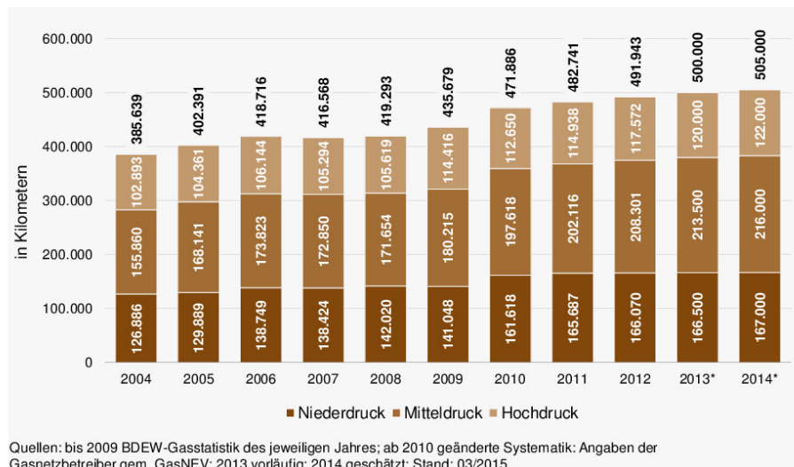
Bild 11 Entwicklung der Gasnetztlänge in Deutschland (Quelle: BDEW 3/2015).
