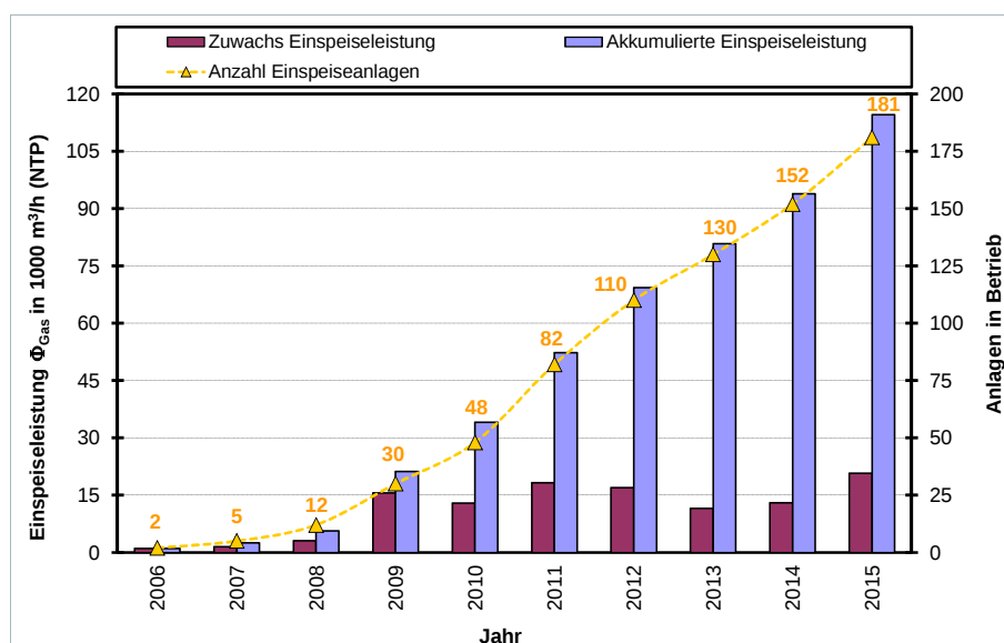
Bild 14 Entwicklung der Biogaseinspeisung in Deutschland (Daten aus [48]).
