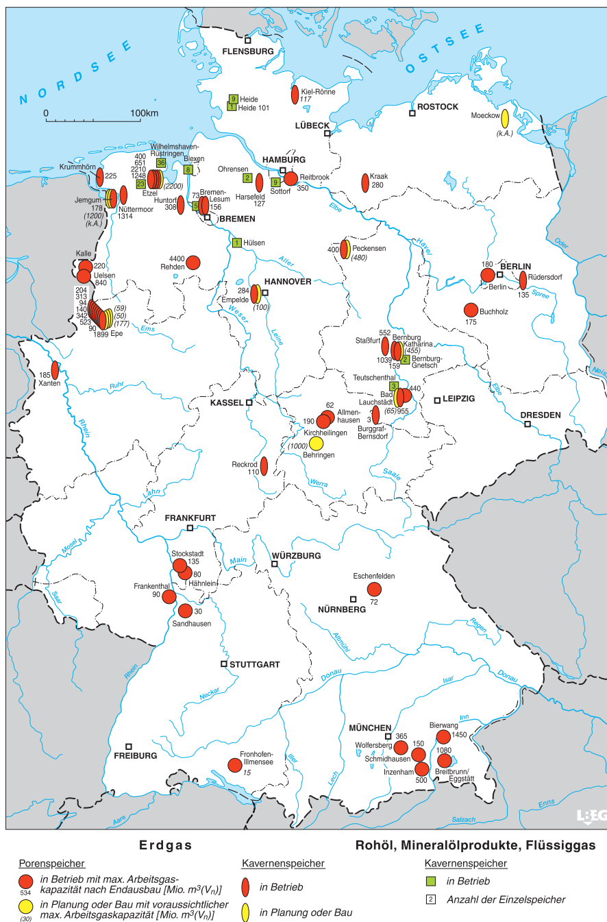
Bild 5 Erdgas-Untertage-speicher in Deutschland [16].
