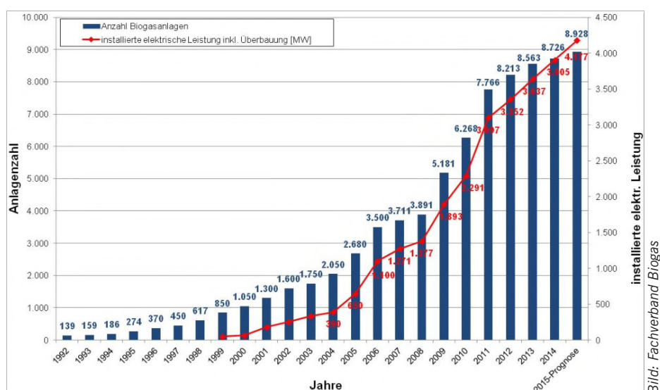
Bild 12 Entwicklung des Biogasanlagen-Bestandes.
